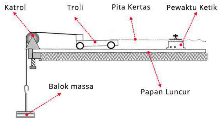
Gambar 3.3 Skema praktikum gerak lurus berubah beraturan
