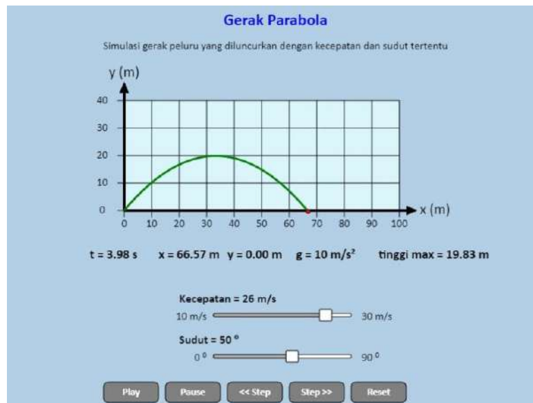
Gambar 3.5 Elemen interaktif pada simulasi gerak parabola
