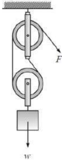
Gambar 10.5 Simulasi katrol ganda.
