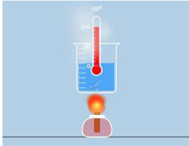
Gambar 11.2 Rancangan simulasi pengukuran panas
