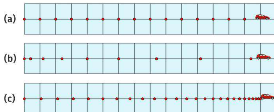
Gambar 9.2 Hasil Simulasi
