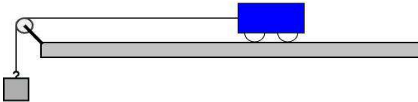
Gambar 9.3 Model simulasi GLBB dengan beban massa
