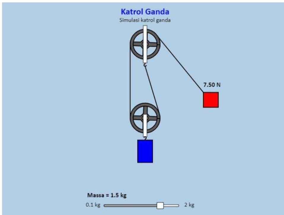
Gambar 10.6 Hasil tutorial simulasi katrol ganda
