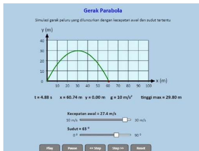
Gambar 9.5 Hasil simulasi gerak parabola
