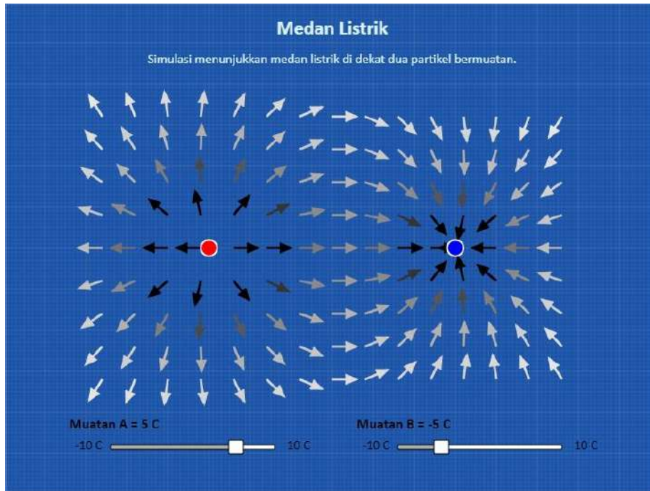
Gambar 12.2 Hasil tutorial medan listrik
