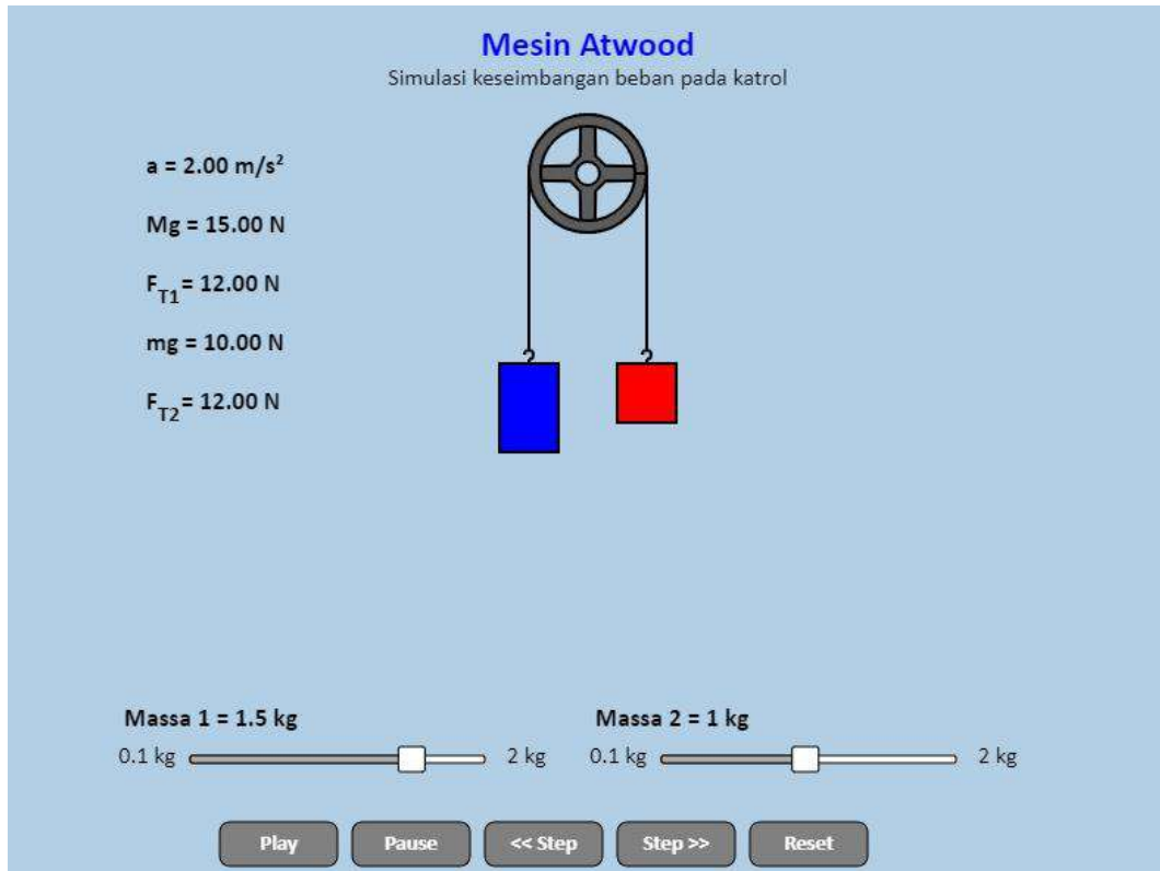
Gambar 10.3 Hasil tutorial simulasi mesin Atwood
