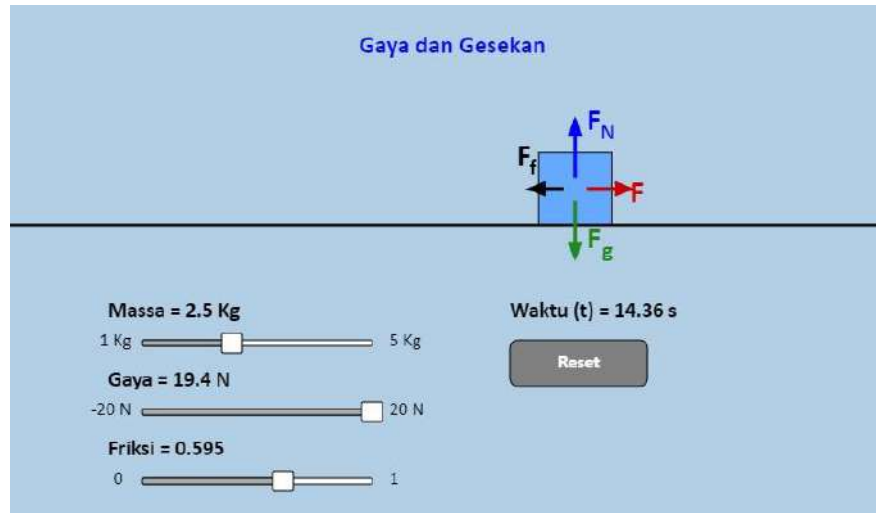
Gambar 10.1 Hasil tutorial Simulasi Hukum Newton
