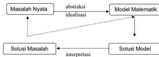
Gambar 3.1 Pemodelan matematika
