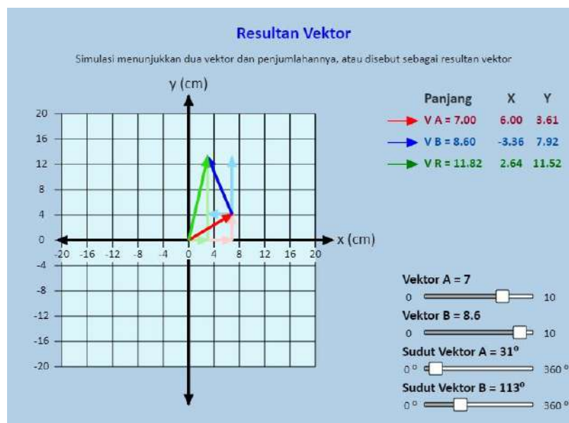
Gambar 8.1 Hasil tutorial penjumlahan vektor
