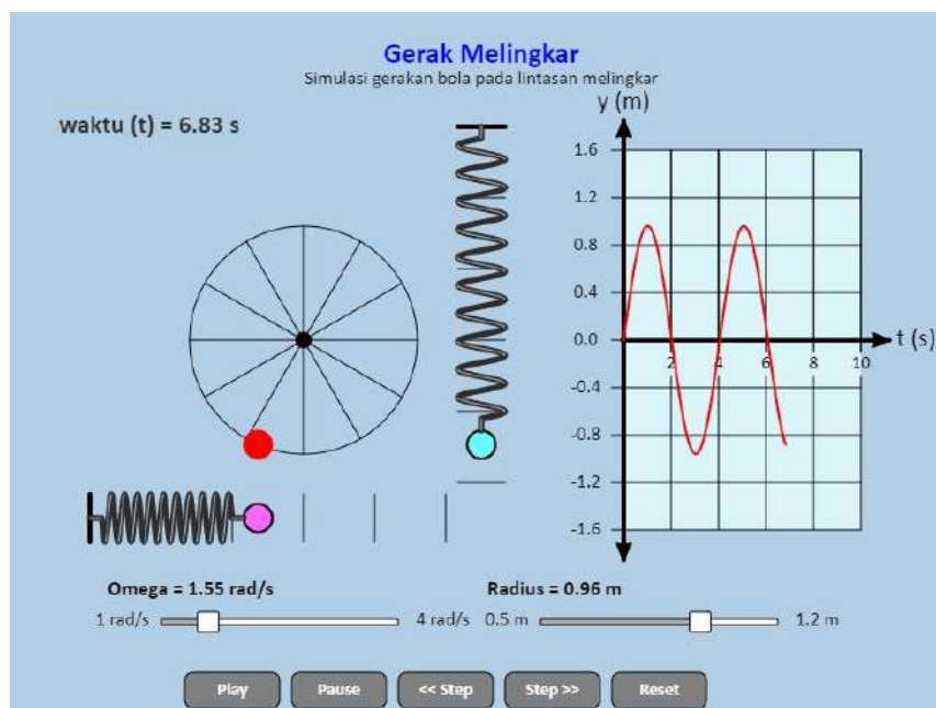
Gambar 9.6 Hasil simulasi gerak melingkar
