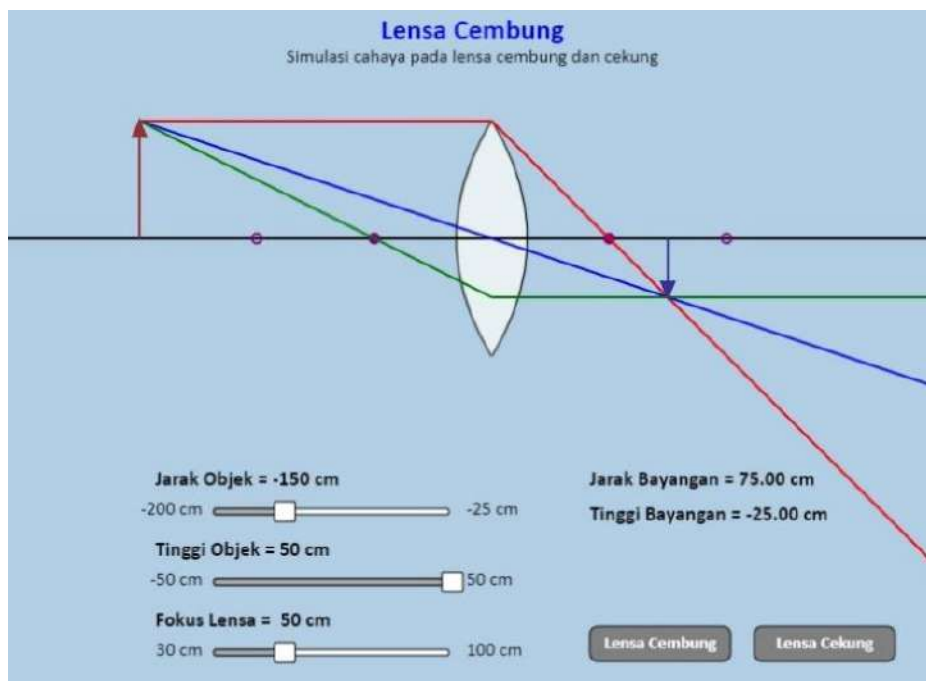
Gambar 12.1 Hasil tutorial lensa
