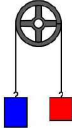
Gambar 10.2 Simulasi keseimbangan beban pada mesin Atwood.
